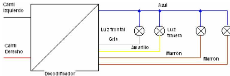
Figura 4. Conexión con + común
